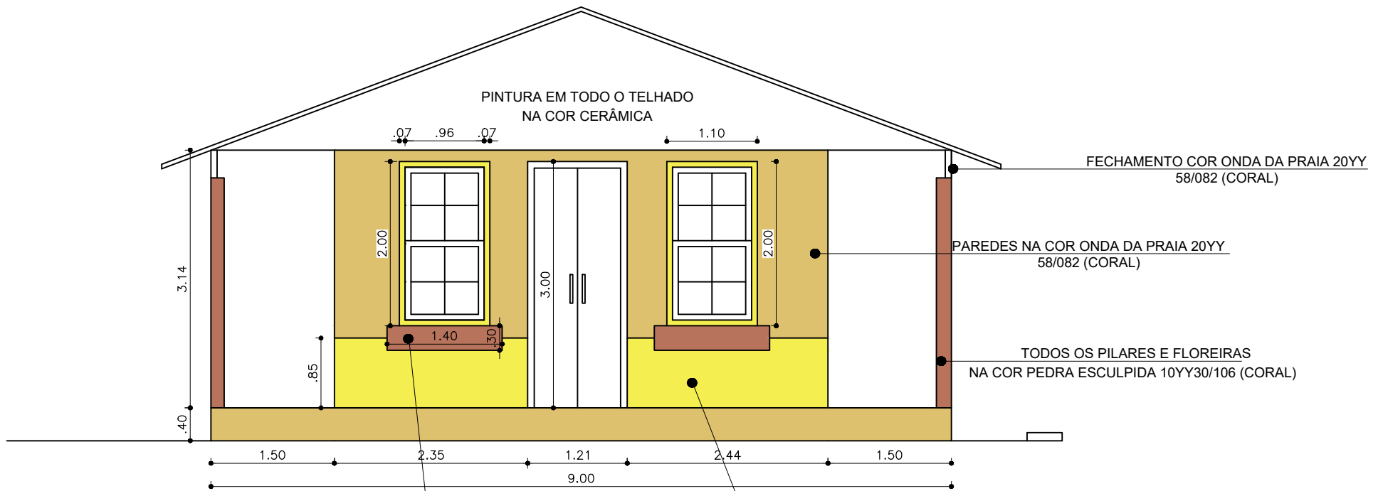
VISTA A- FACHADA PRINCIPAL
